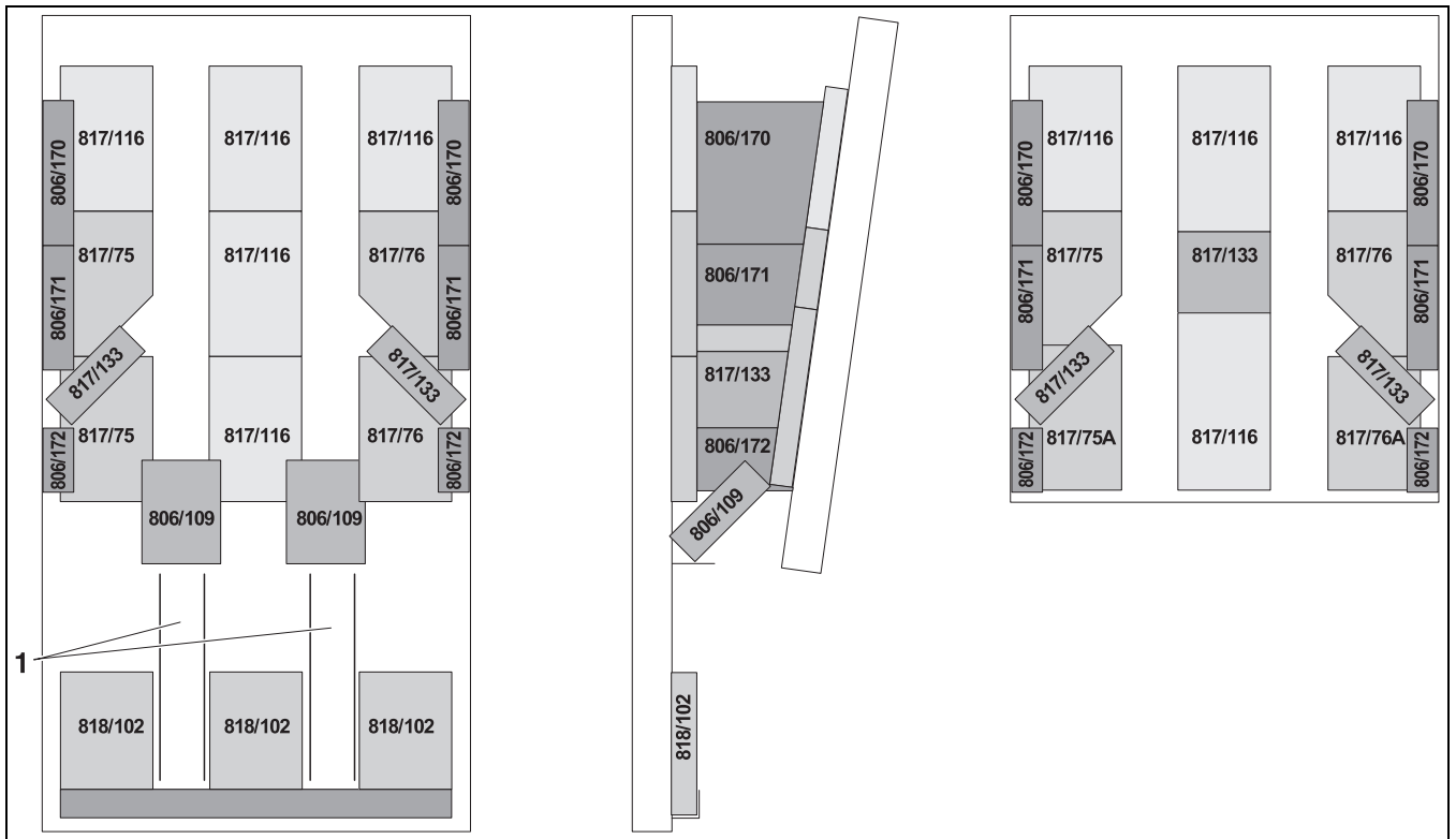
sl. 18 Postavljanje šamotnih ploča kod tipa K 32-1 S/SW 62
